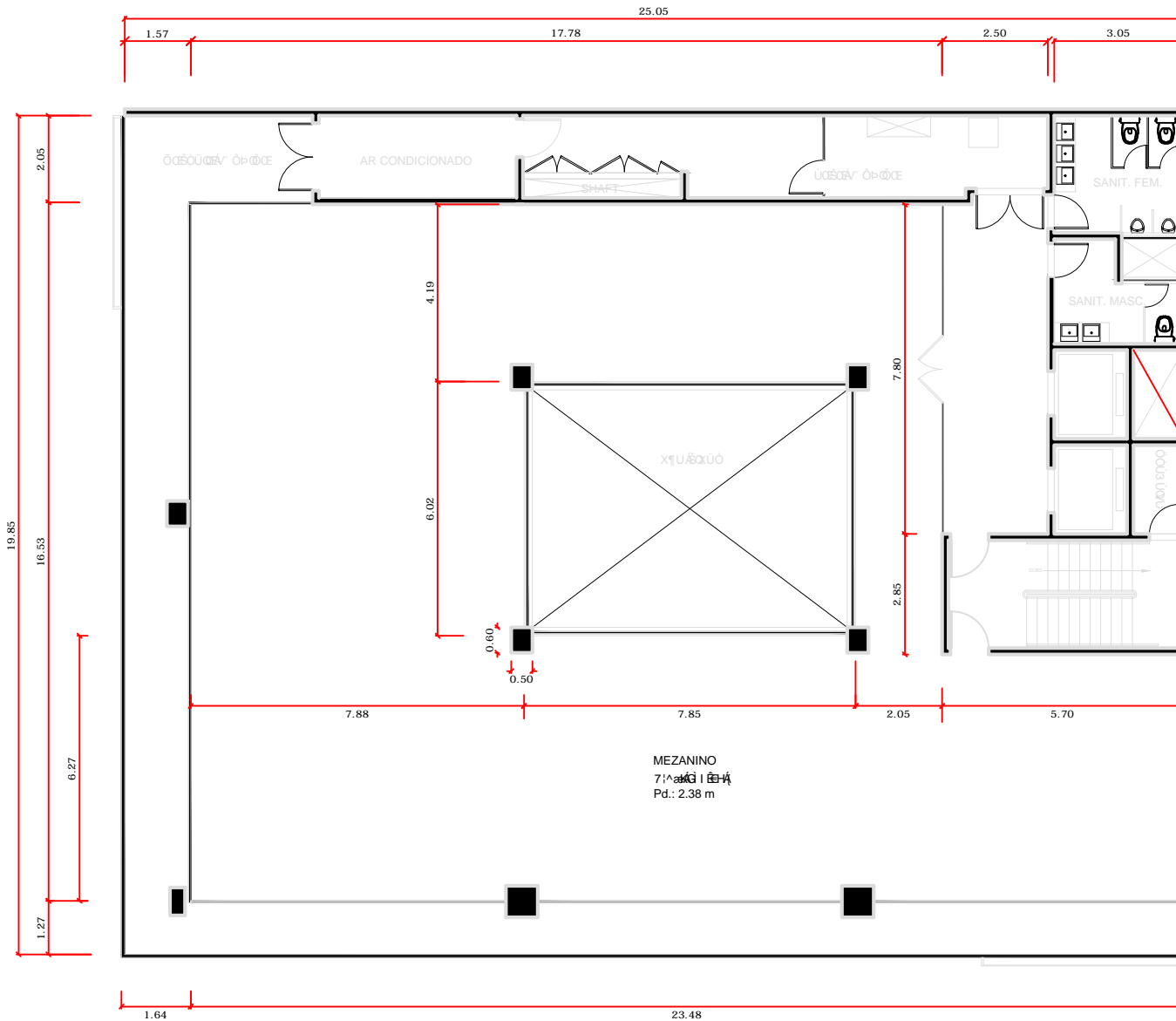
PLANTA BAIXA MEZANINO
